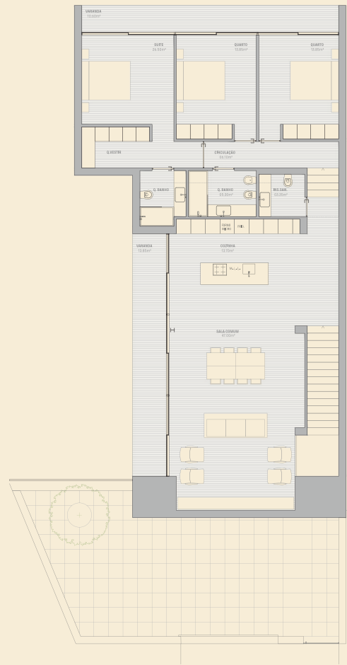
Planta Piso 2
